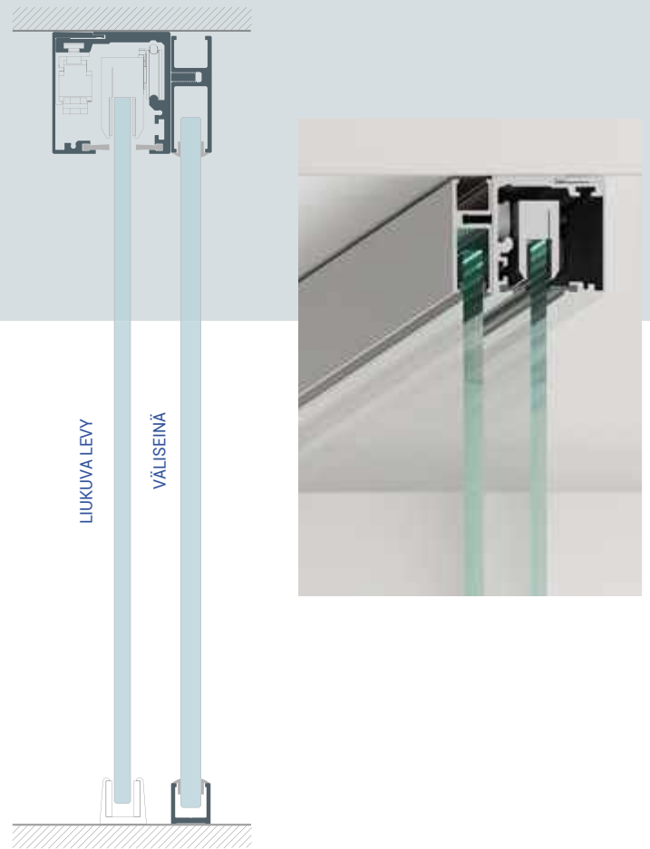
■ Leikkaus 4-4
