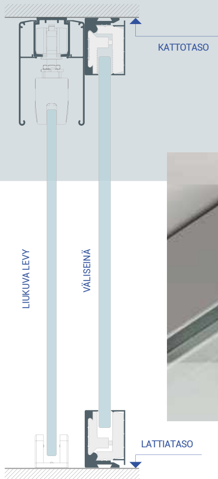
■ Leikkaus 3-3
